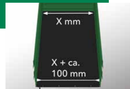
A kúpos kialakítású platólemez garantálja a rakomány üritését
