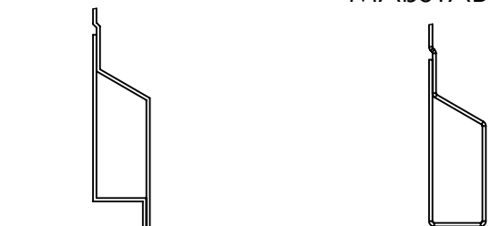
DETAIL G MAßSTAB 1 : 4
